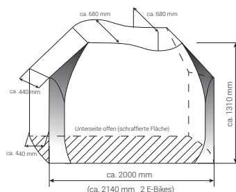
Universal Zwoo - 2 Räder
