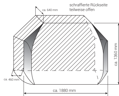
für bis zu 3 Räder
