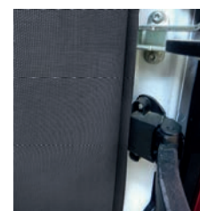
Magnetleiste in Türfalz.
