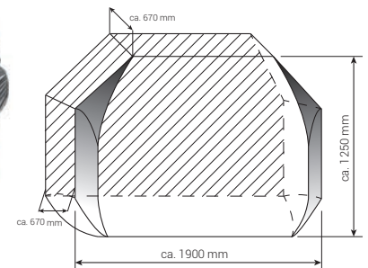
Ansicht mit geschlossenen Hecktüren
